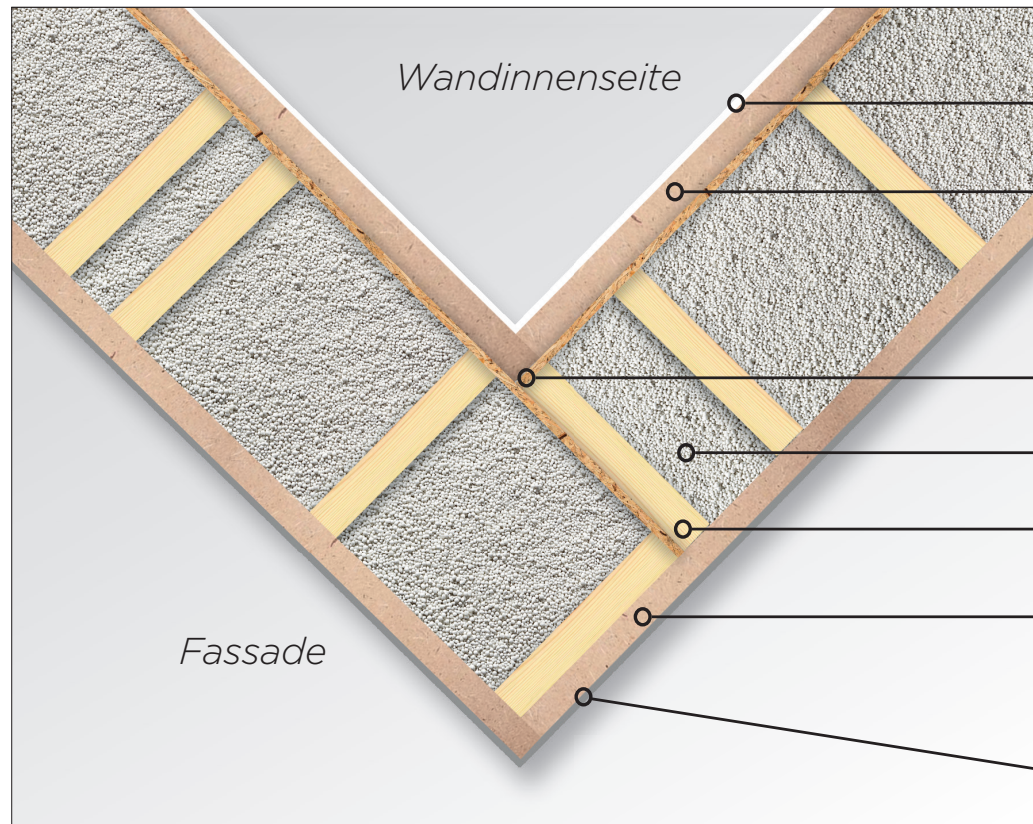
Schematischer Wandaufbau (Eckkonstruktion)
