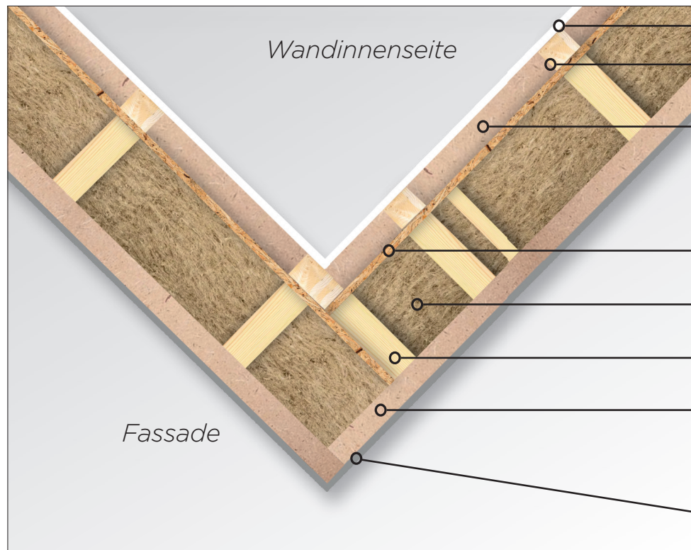
Schematischer Wandaufbau (Eckkonstruktion)
